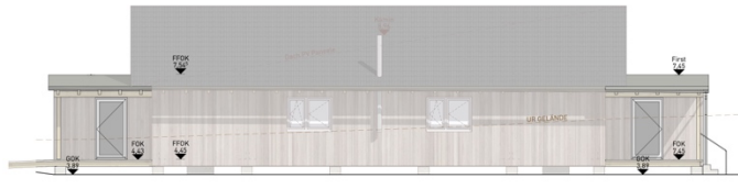
Gartenhütte Ostansicht M1:100
